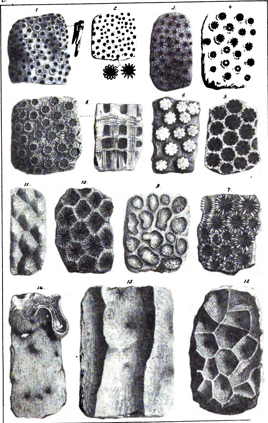
Quenstedt, Jura.
